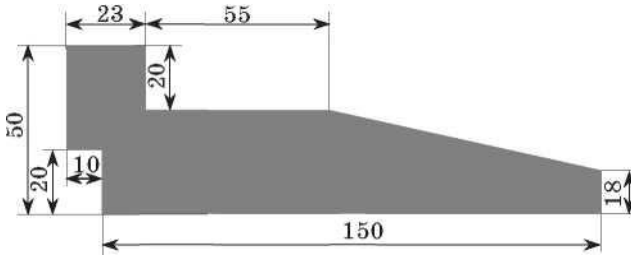
Грудна фігура (мішень № 6а)
