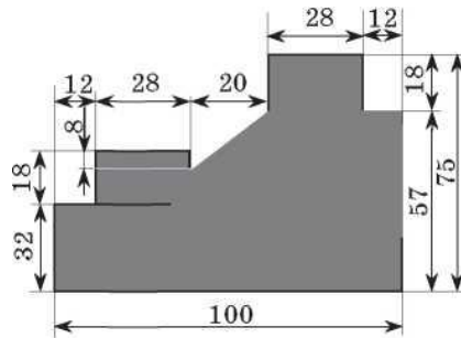
Кулеметна обслуга (мішень № 10а)
