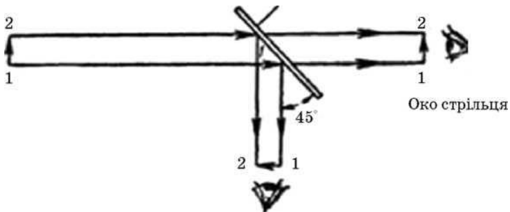
Мал. 9. Автомат з бічним склом
