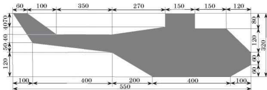
Вертоліт (мішень № 25а)
