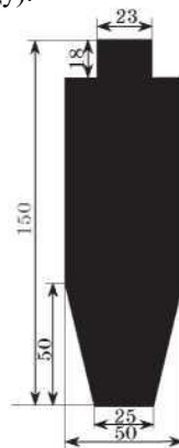
Ростова фігура (мішень № 8)
