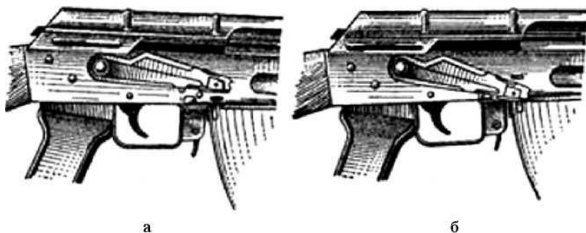
Мал 5. Установка перевідника
