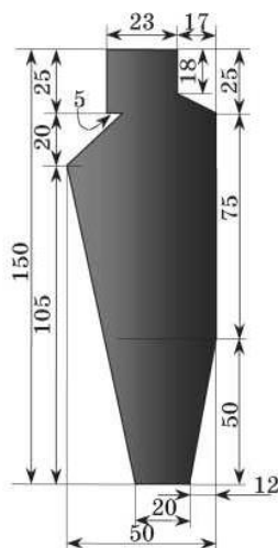
Ростова фігура (мішень № 8а)
