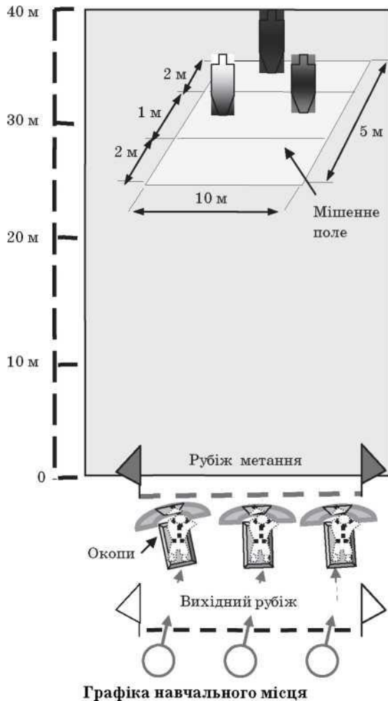
Графіка навчального місця
