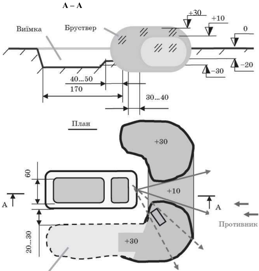
Нарощування брустверу на всю довжину окопу для ведення флангового вогню Окоп для стрільби із автомата лежачи
